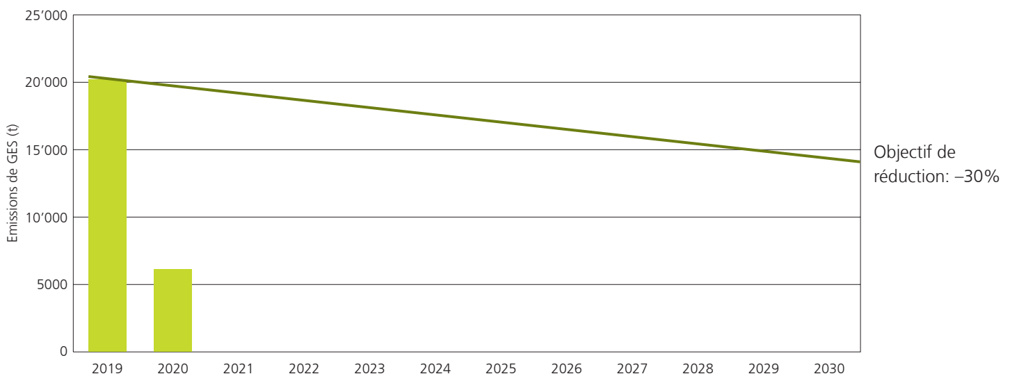
Figure 4: Évolution des émissions de GES dues aux voyages en avion depuis 2019.
