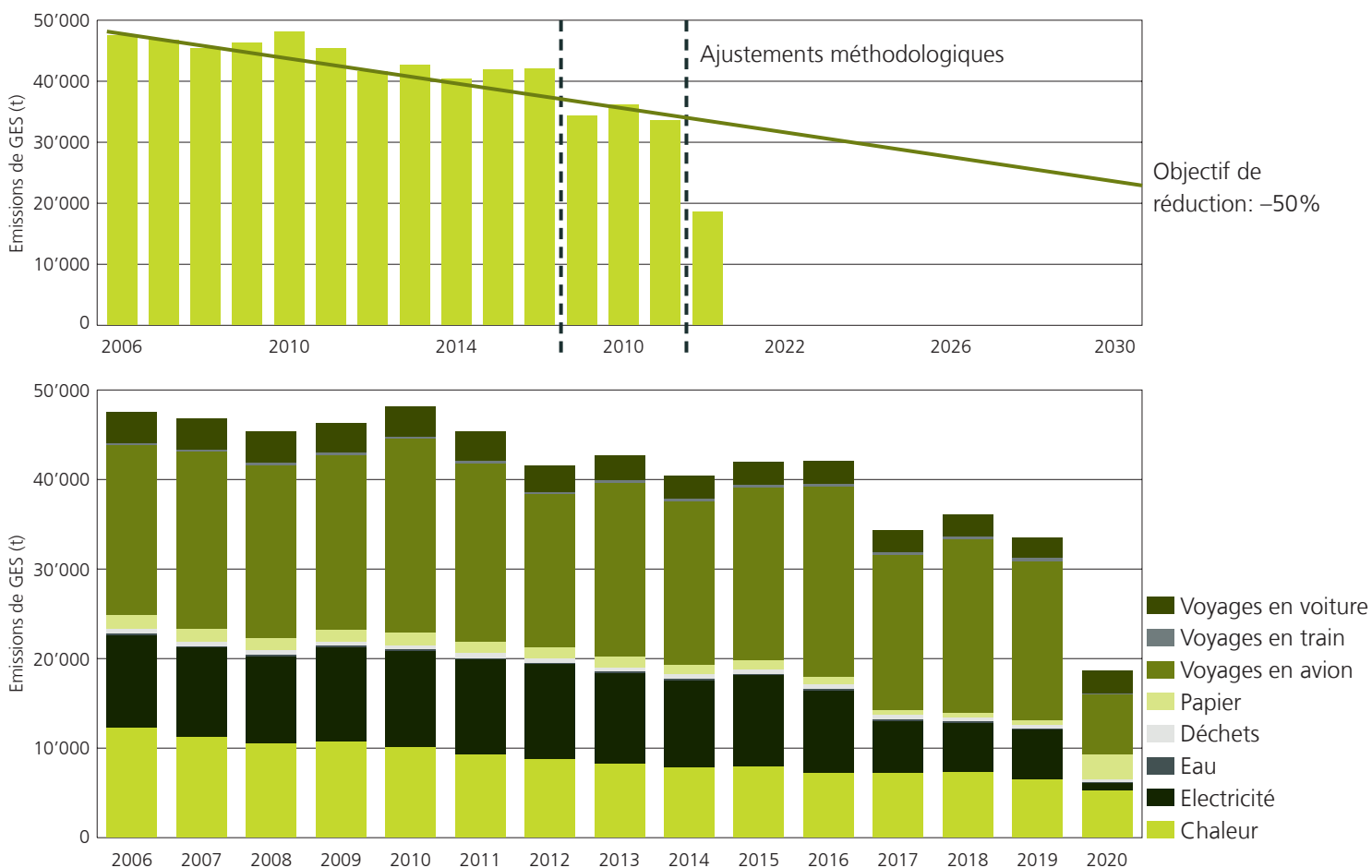
Figure 3: Évolution des émissions de GES depuis 2006
